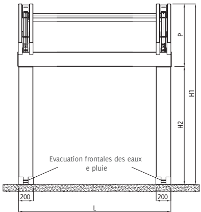
Vue Frontale
